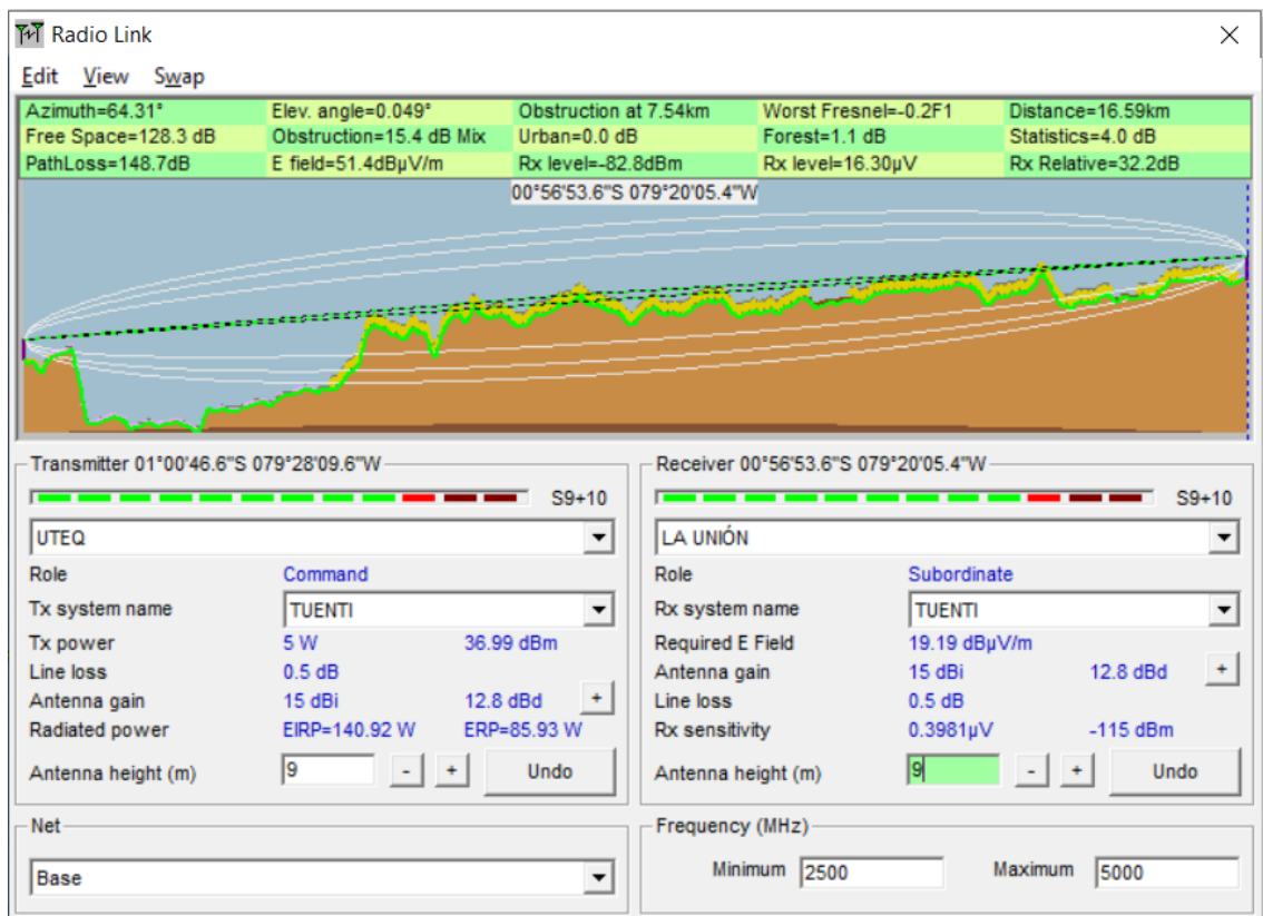
Ilustración 8. Radio Link
